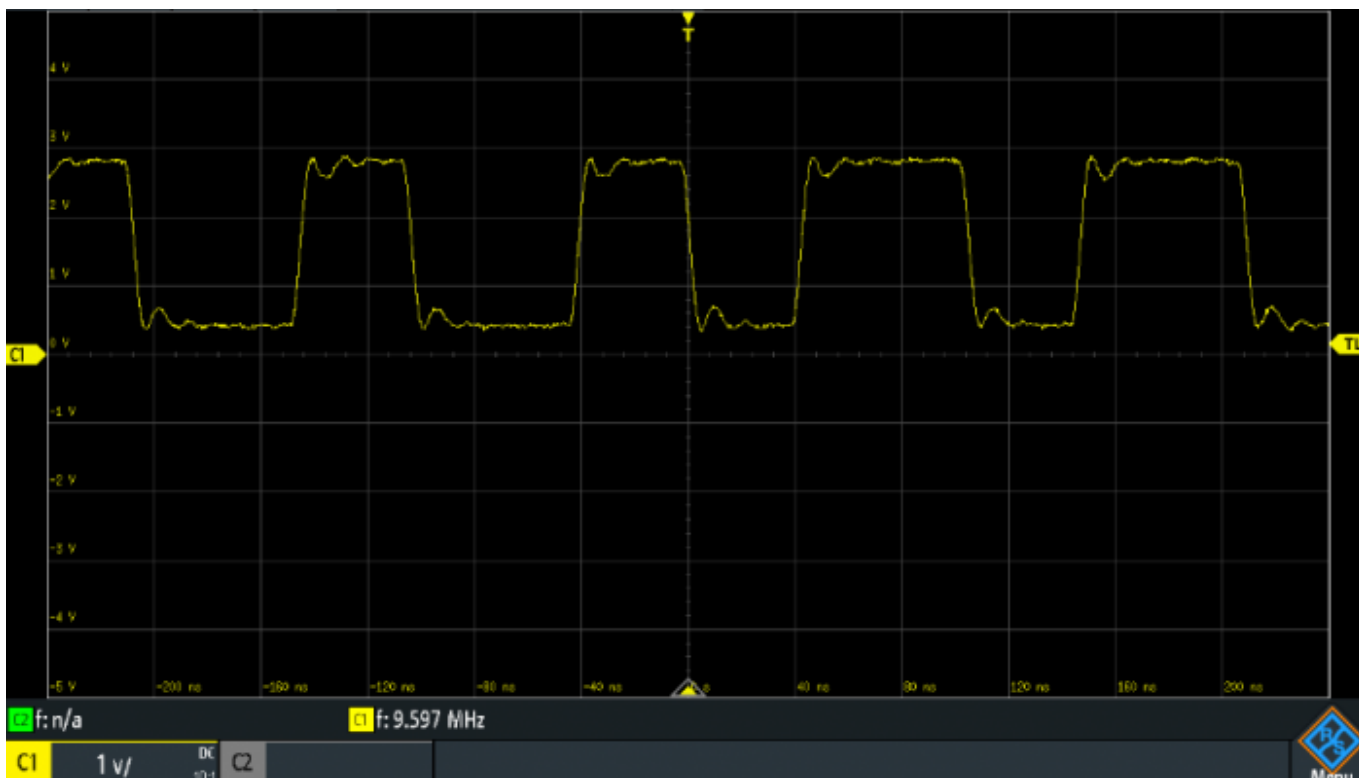
10 MHz Ausgangssignal des MAX8Q
